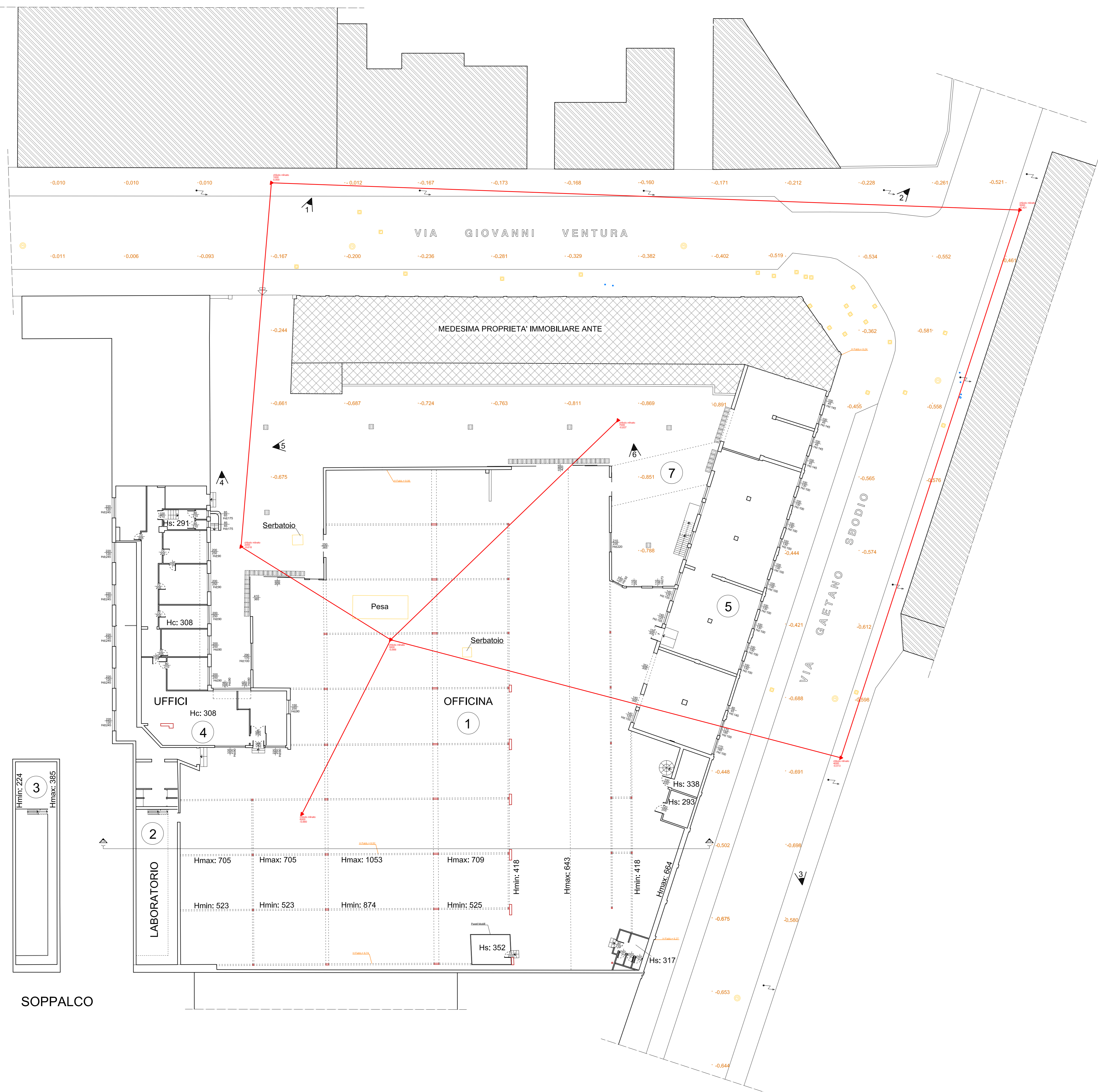
PLANIMETRIA GENERALE
